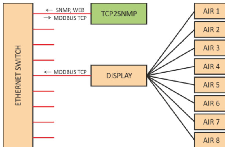
Blokové schéma zapojení
